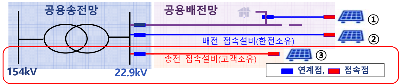
[그림 1] 22.9kV로 송전용 전기설비를 이용하는 경우(예시)
